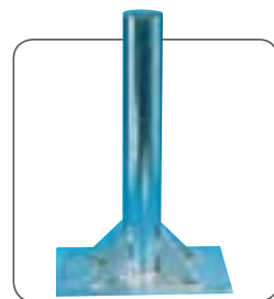
Base pletina en acero galvanizado. Medidas de la base: 30 x 30 cm. Altura: 60 cm. Peso: 7 kg.
