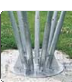
Base ramo Tubo de acero galvanizado. Para mástiles de ø 65 mm.
