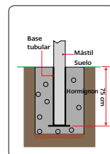
Base empotrada (en aluminio)
