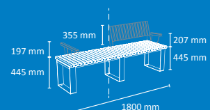
Plano detalle
